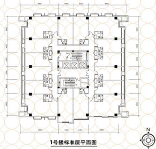
1#楼标准层平面图
